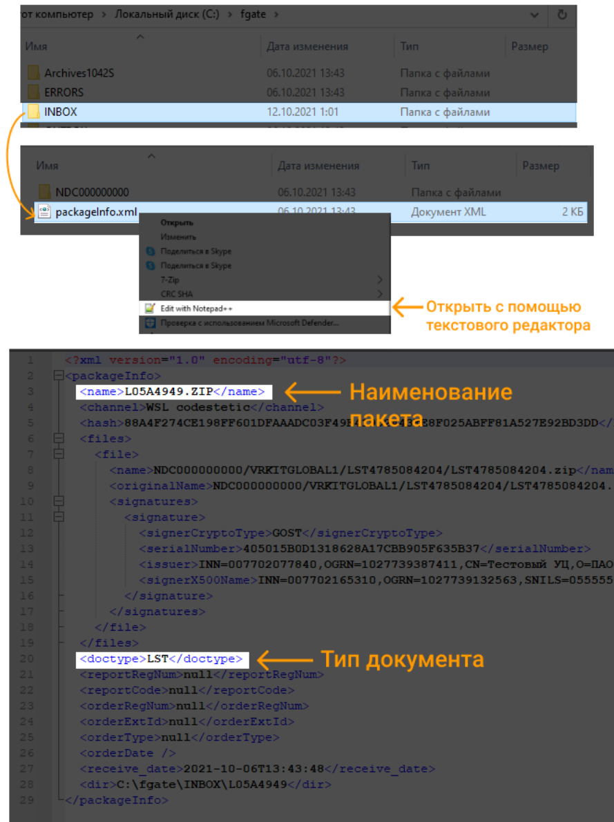
Рисунок 130. Просмотр информации в packageInfo.xml
