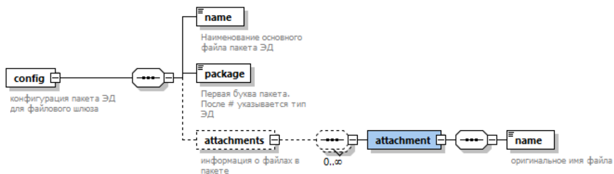
Рисунок 18. Структура файла config.xml
