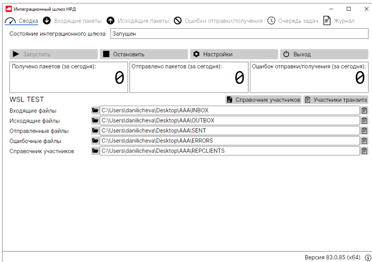
Рисунок 2. Вид ИШ при первом запуске
