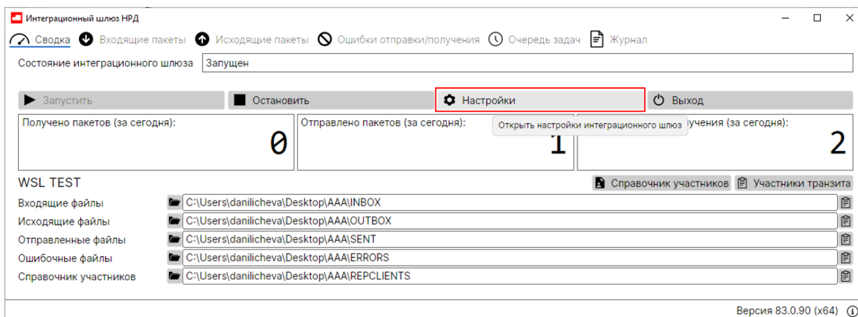
Рисунок 12. Настройки
