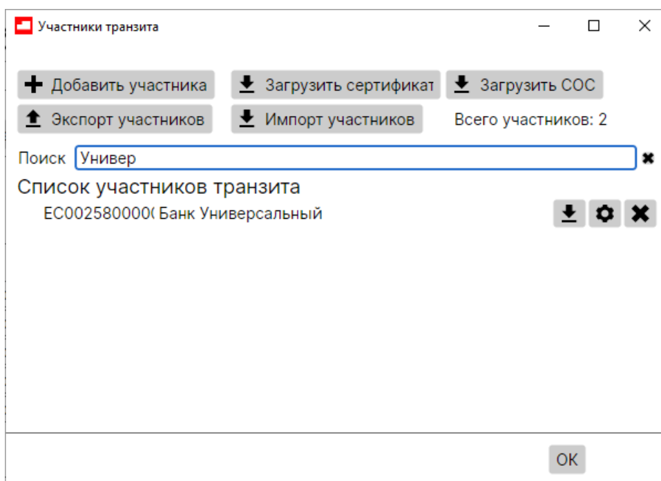
Рисунок 23. Поиск участника
