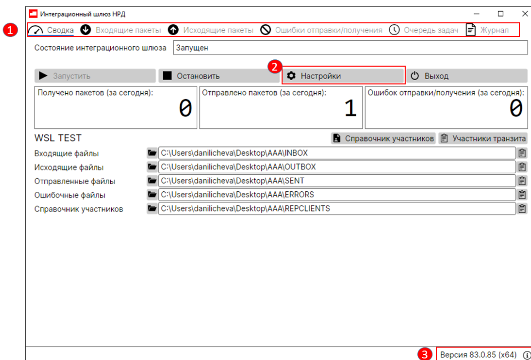
Рисунок 3. Интерфейс ИШ
