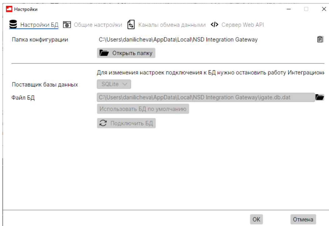
Рисунок 13. Настройки
