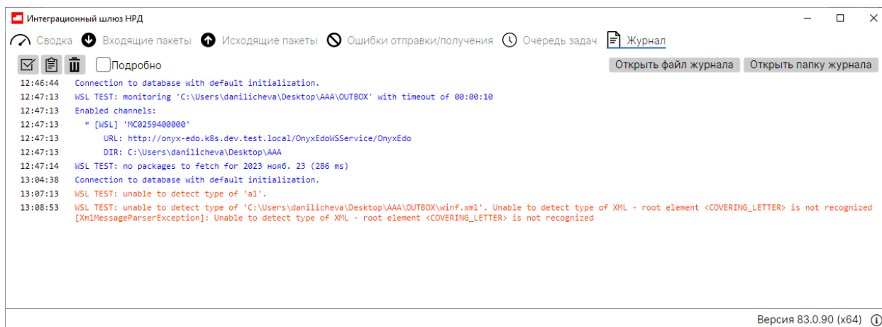
Рисунок 10. Журнал
