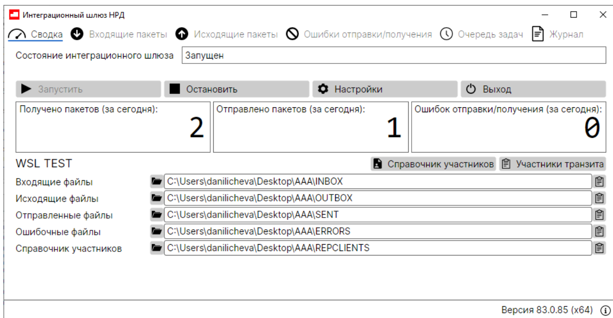
Рисунок 4. Сводка
